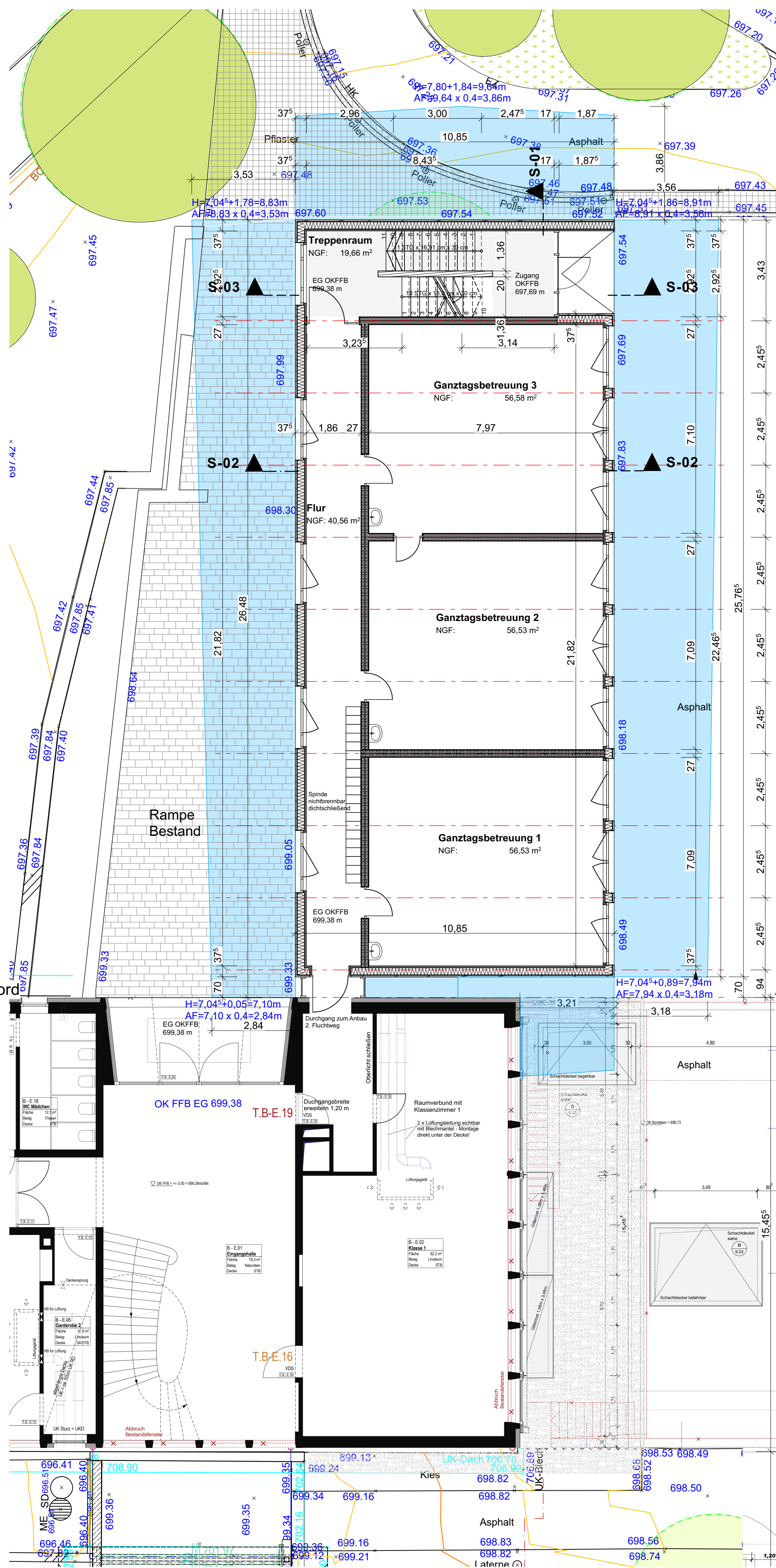
Grundriss Erdgeschoss
