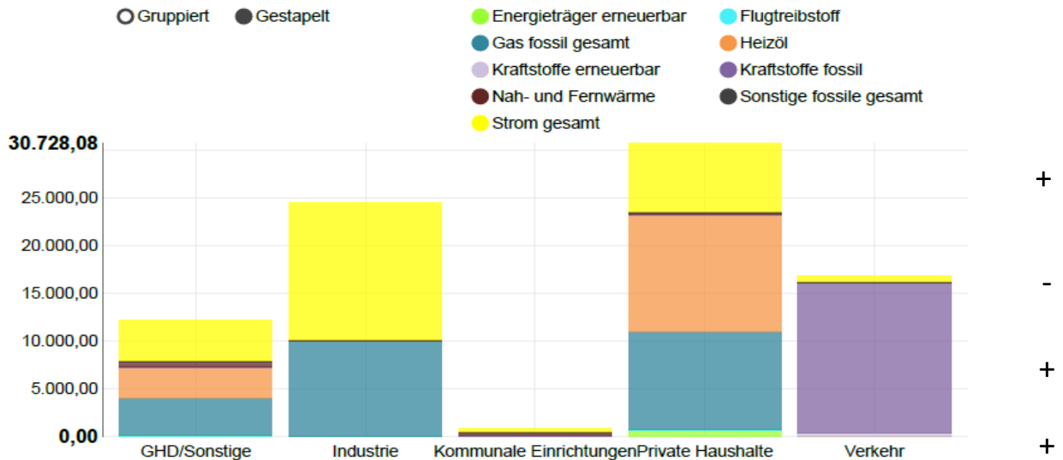
Abbildung 2: Treibhausgasemissionen in t CO 2 -Äquivalente nach Sektoren und Energieträgern für 2021
