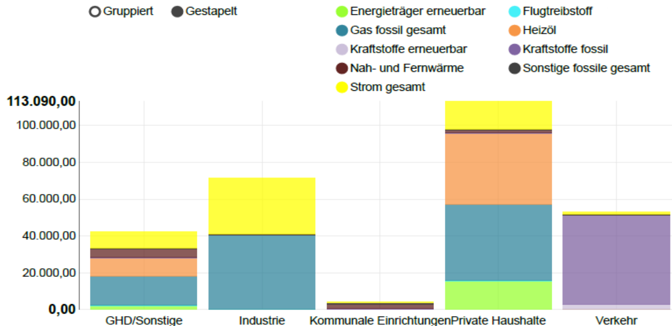
Abbildung 1: Endenergieverbrauch in MWh nach Sektoren und Energieträgern für 2021
