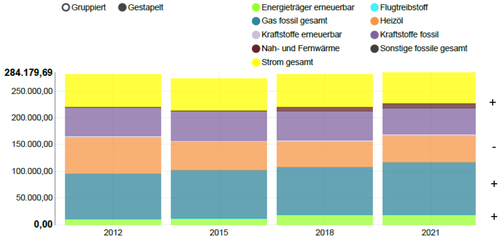
Zeitreihen - Endenergieverbrauch in MWh nach Energieträgern
